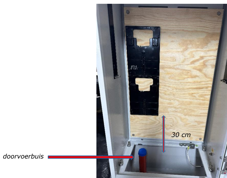
Voorbeeld doorvoerbuis
