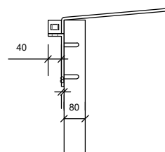
doorsnede detail A luik is af te sluiten d.m.v. hangslot
