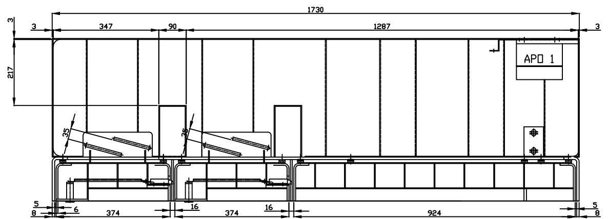
DOORSNEDE D-D
