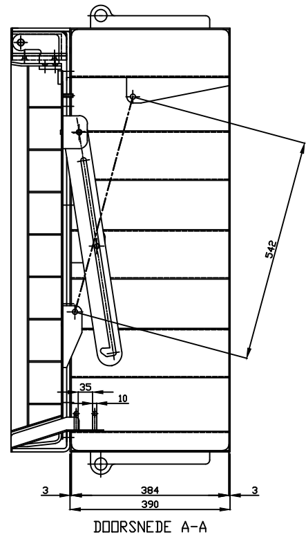
DOORSNEDE A-A
