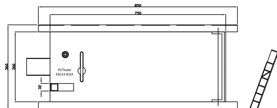
BOVEN AANZICHT MET GESLOTEN DEKSEL
