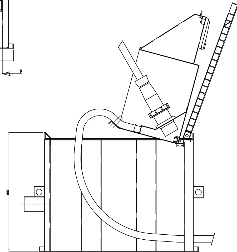
DOORSNEDE B-B MET GEOPEND DEKSEL EN LUCHTKLOK
