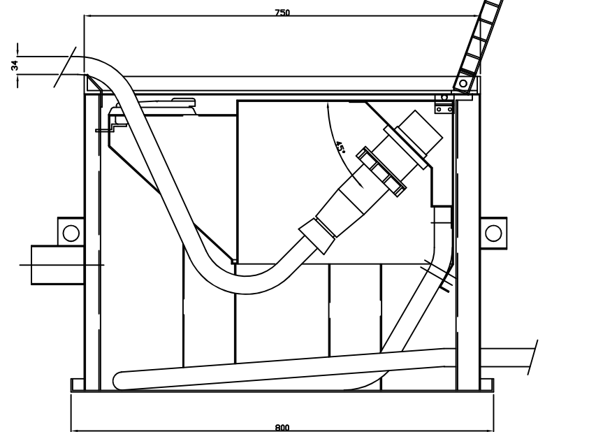
DOORSNEDE B-B MET GEOPEND DEKSEL
