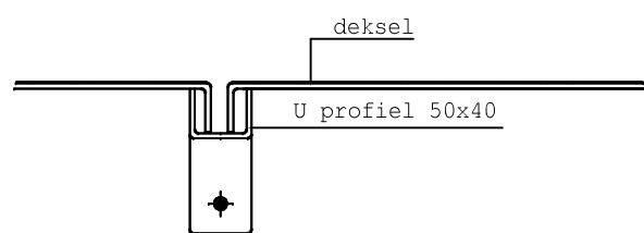
doorsnede detail C ondersteuning en afsluiting tussen deksels
