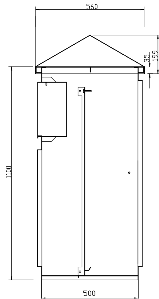
DOORSNEDE A-A
