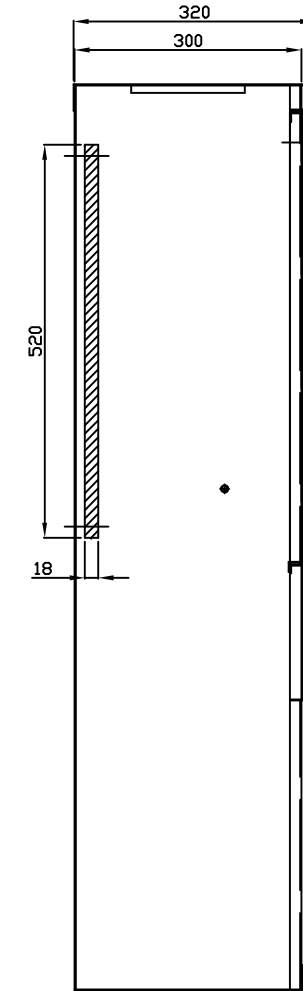
DOORSNEDE A-A
